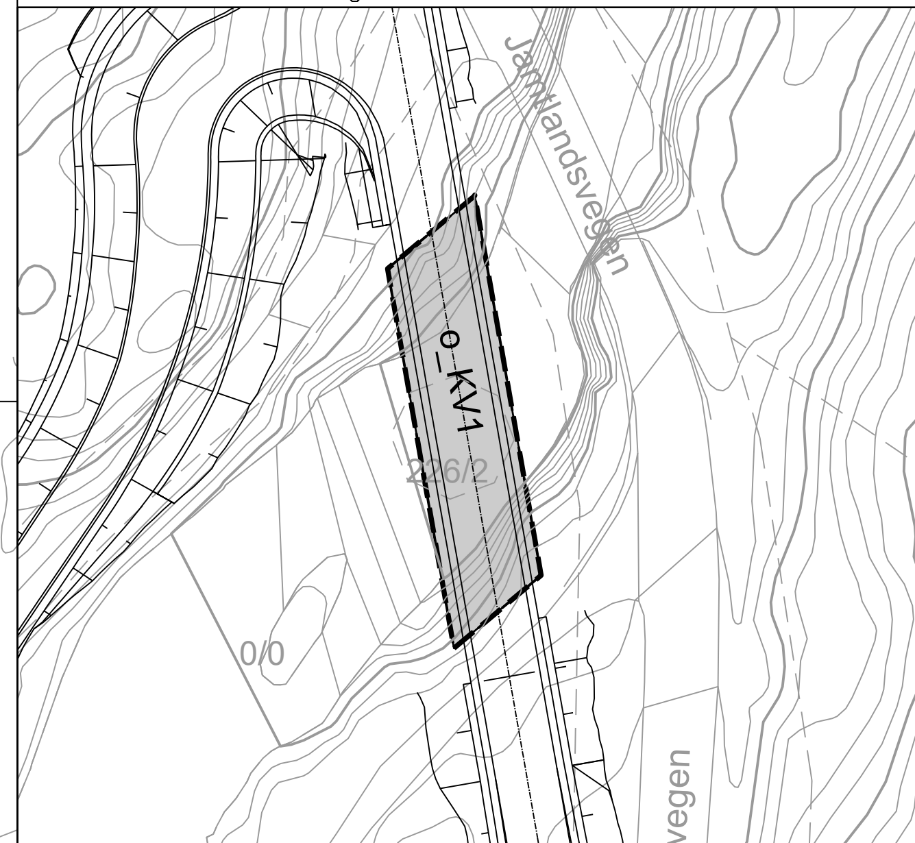
Vertikalnivå 3 - Over grunnen (bru) 1:500m
