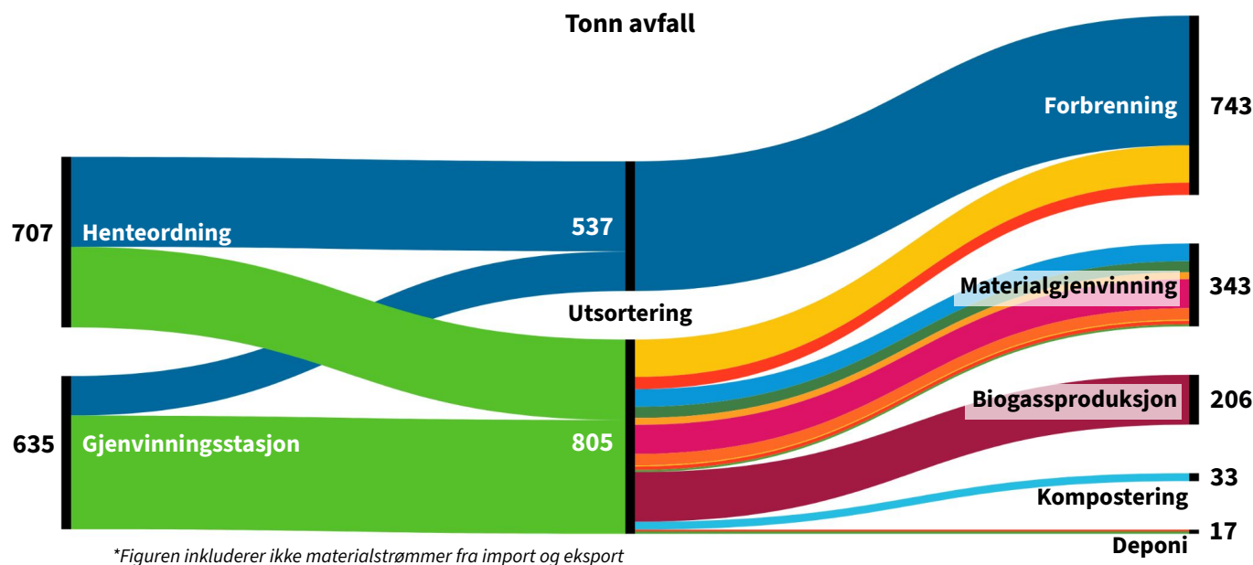
Utsnitt av verdikjeden med kvantifiserte strømmer for avfall i Overhalla kommune (2022)
