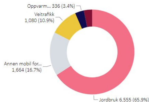
Utslipp (tonn CO 2 -ekvivalenter) per sektor i Lierne i 2021
