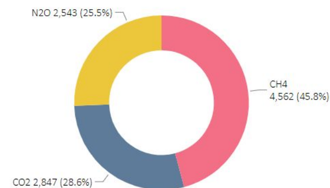
Utslipp (tonn CO 2 -ekvivalenter) i Lierne i 2021 per klimagass
